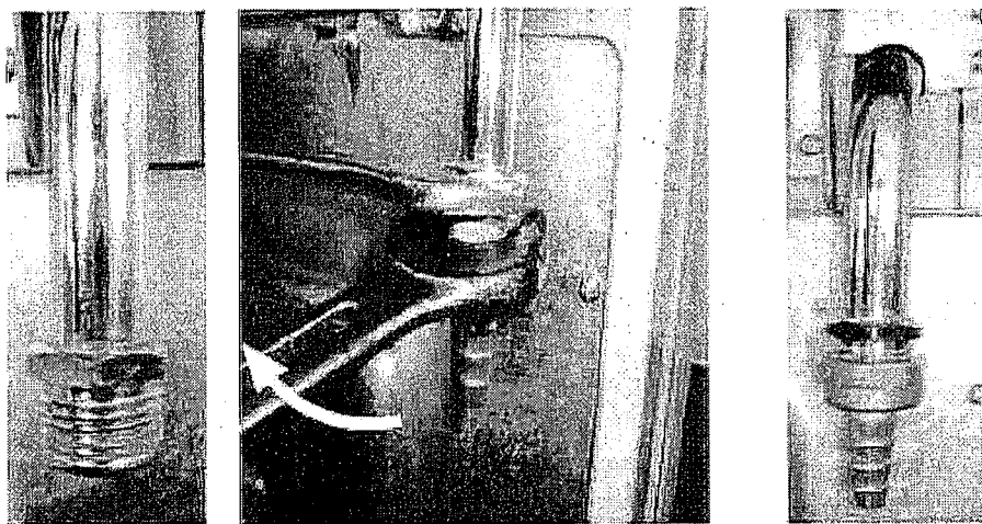
Figure 13 Montage de l'embout gaz butane
